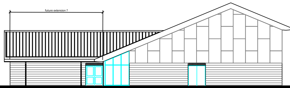
ELEVATION 4
